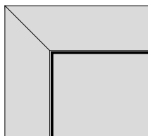
łączenie opasek 45°
