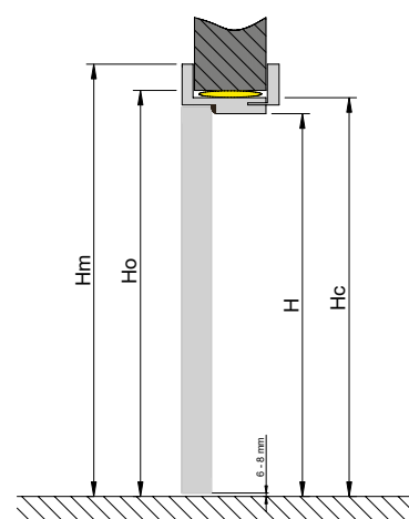
Przekrój pionowy drzwi
