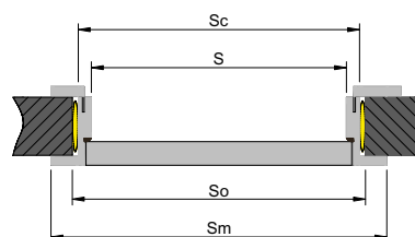
Przekrój poziomy drzwi
