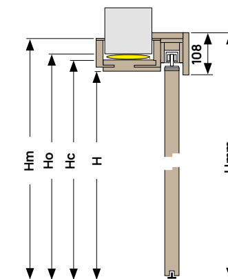
Przekrój pionowy
